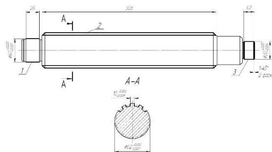
Рисунок 2 – Эскиз вала заднего хода
